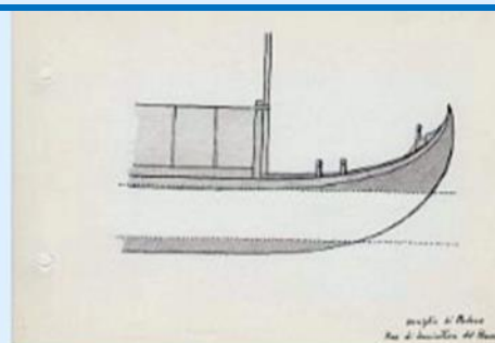
120-Naviglio di Modena - prua di bucintoro del Panaro
