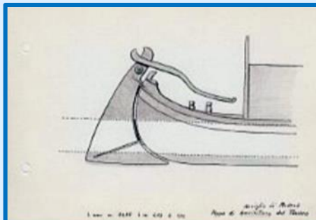
119-Naviglio di Modena - poppa di bucintoro del Panaro
