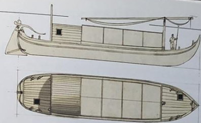
I marinai di Chioggia e della laguna di Venezia, riconoscevano da lontano l'arrivo dei barcai modenesi dalla prua di questa originale imbarcazione.
