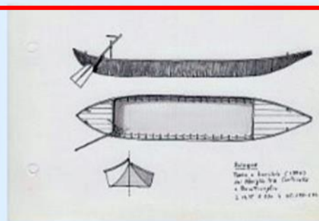
124-Bologna- paron o burchio - 1890 - del Naviglio tra Corticella e Bentivoglio -
