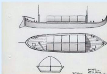
118-Bastardo - poppa di burchio - prua di rascona - Ticino - Po - Panaro
