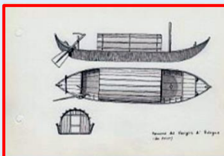
123-Rascona del Naviglio di Bologna - sec. XVIII
