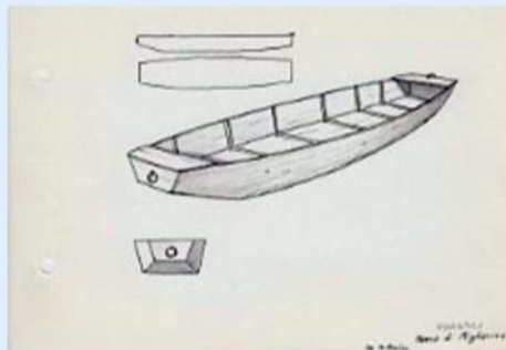
122-Ferrara - Barca di Migliarino - da M. Bonino
