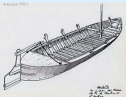
117-Barbota - da modello del Museo del Po di Monticelli d'Orngina
